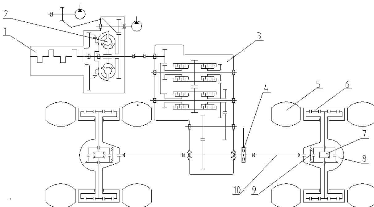
شکل ۴-۱ سیستم محرک
