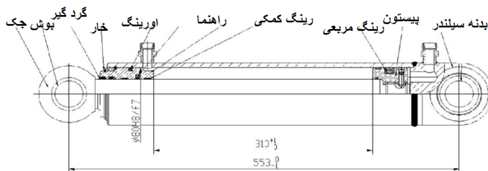
شکل ۴-۶ جک فرمان
