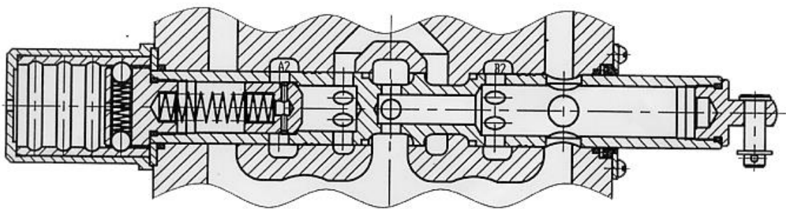
شکل ۱۲-۴ موقعیت بلند کردن بوم در اسپول شیر بوم
