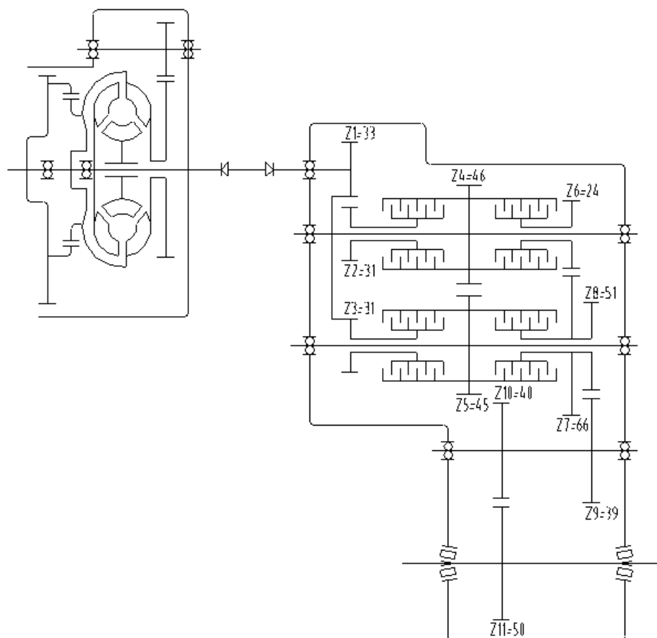
شکل ۲-۴ قسمت های مهم گیربکس
