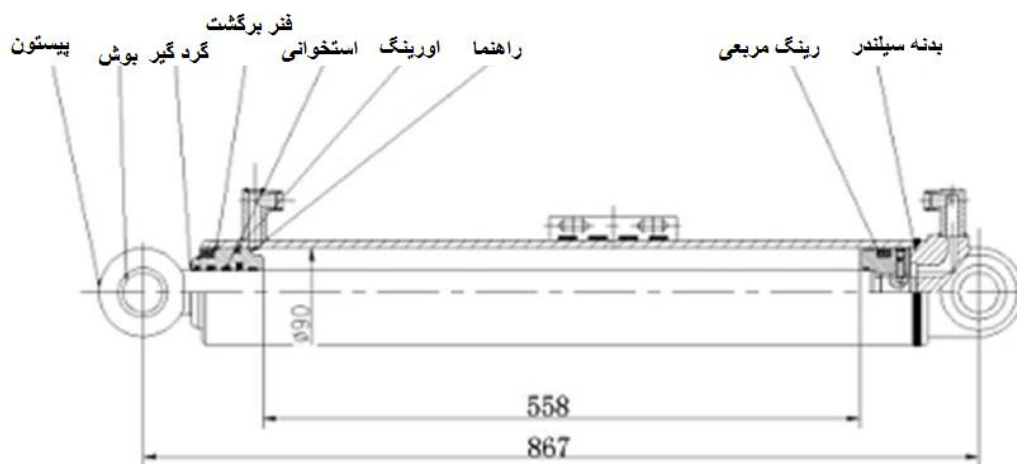
• شکل ۸-۴ جک بوم
