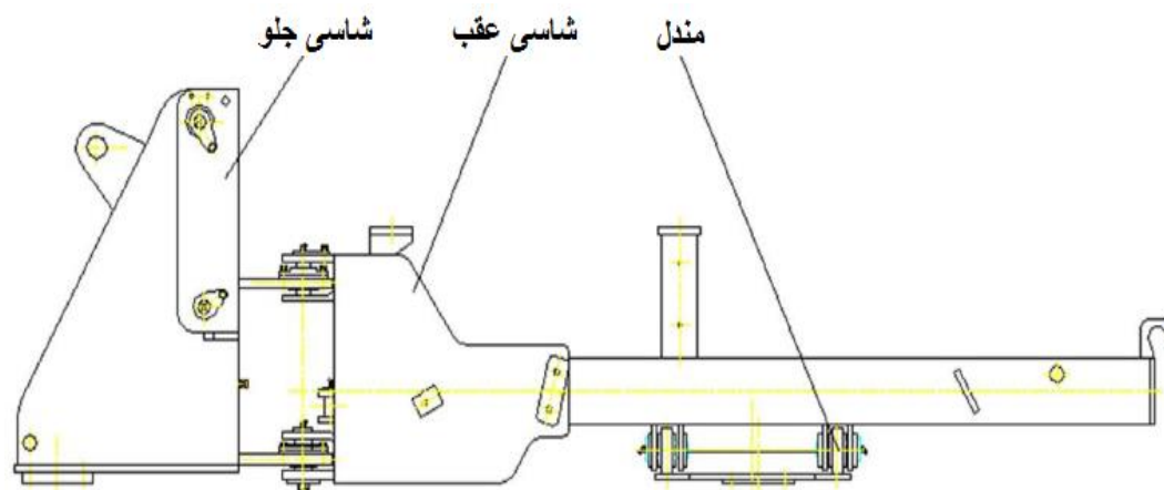
شکل ۲۰-۴ شاسی
