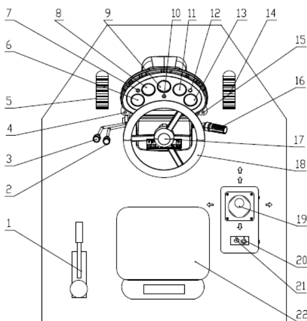
شکل ۱-۳ داشبورد و مکانیزمهای کنترلی
