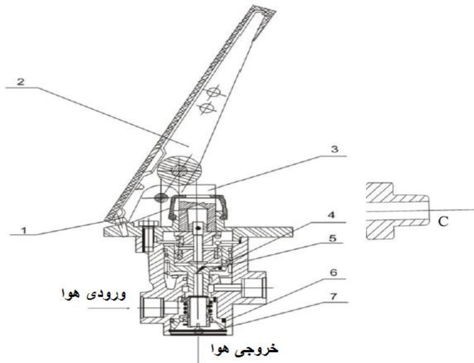
شکل ۲۳-۴ پدال ترمز
