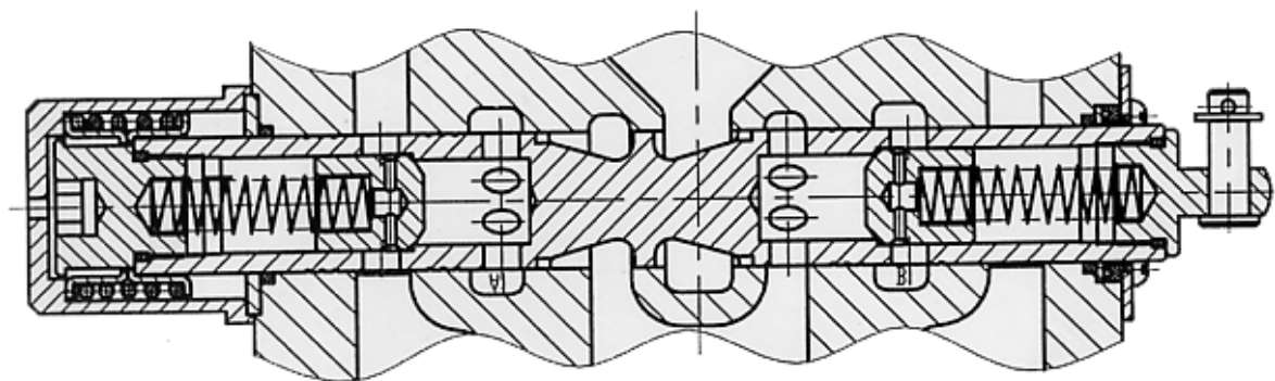
شکل ۱۶-۴ تخلیه باکت
